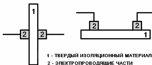
Рис. 5. Два варианта взаимного расположения электропроводящих частей и твердого изоляционного материала с весьма отличающимися диэлектрическими свойствами
