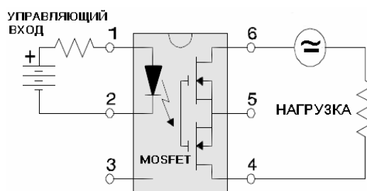
Рис. 1. Принципиальная схема твердотельного реле на MOSFET транзисторах, предназначенного для коммутации и переменного и постоянного тока
