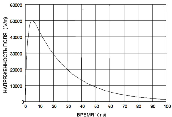
Рис. 3. Форма компонента ЭМИЗ в соответствии со стандартами IEC 61000-2-9, IEC 61000-2-10, IEC 61000-2-11 и MIL-STD-461F.
