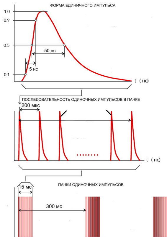
Рис. 5. Electrical Fast Transient (EFT) – быстрый импульс (IEC 61000-4-4).
