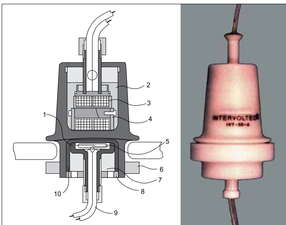
Рис. 3. Реле с регулируемым порогом срабатывания с герконом, расположенным вне катушки, продольная ось которого образует угол с продольной осью катушки: 1 — пластмассовая капсула грибовидной формы с гнездом для геркона; 2 — заливочный эпоксидный компаунд полости корпуса с катушкой; 3 — катушка; 4 — ферромагнитный сердечник; 5 — геркон; 6 — гайка; 7 — заливочный эпоксидный компаунд поворотного корпуса с герконом; 8 — гайка-фиксатор поворотного корпуса; 9 — выводы геркона; 10 — поворотный корпус геркона
