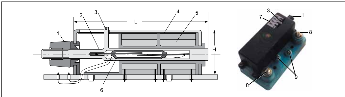
Рис. 2. Герконовое реле с регулируемым порогом срабатывания с аксиальным расположением геркона и катушки и с соосным перемещением геркона: 1 — вращающаяся ручка настройки; 2 — пластмассовая перемещающаяся деталь с запрессованным в нее герконом; 3 — указатель положения геркона; 4 — ферромагнитный экран; 5 — катушка с обмоткой; 6 — геркон; 7 — шкала; 8 — выводы обмотки; 9 — выводы геркона
