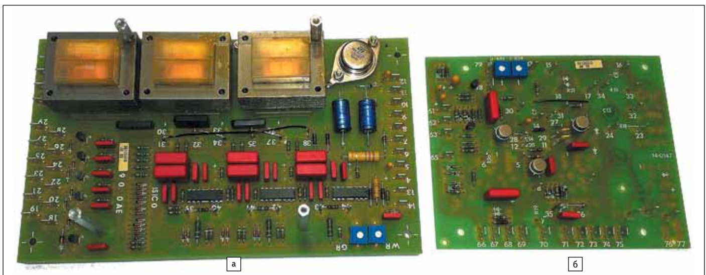
Рис. 5. Два модуля блока управления тиристорами ВЗПА, разработанные и выпускавшиеся в массовом количестве с 70-х годов прошлого столетия компанией АЕГ:
