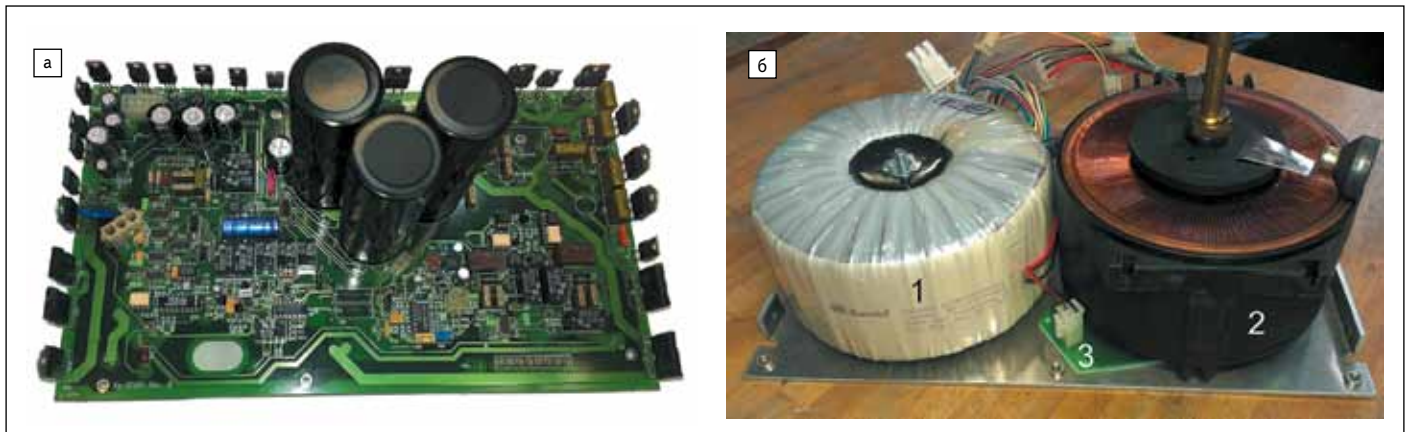
Рис. 4. Устройство В10Е: а) электронный блок; б) силовой блок:
